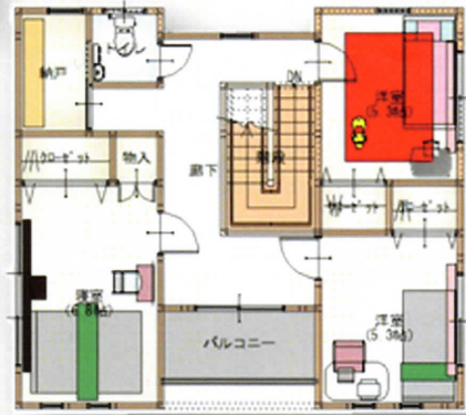
2F 平面図
